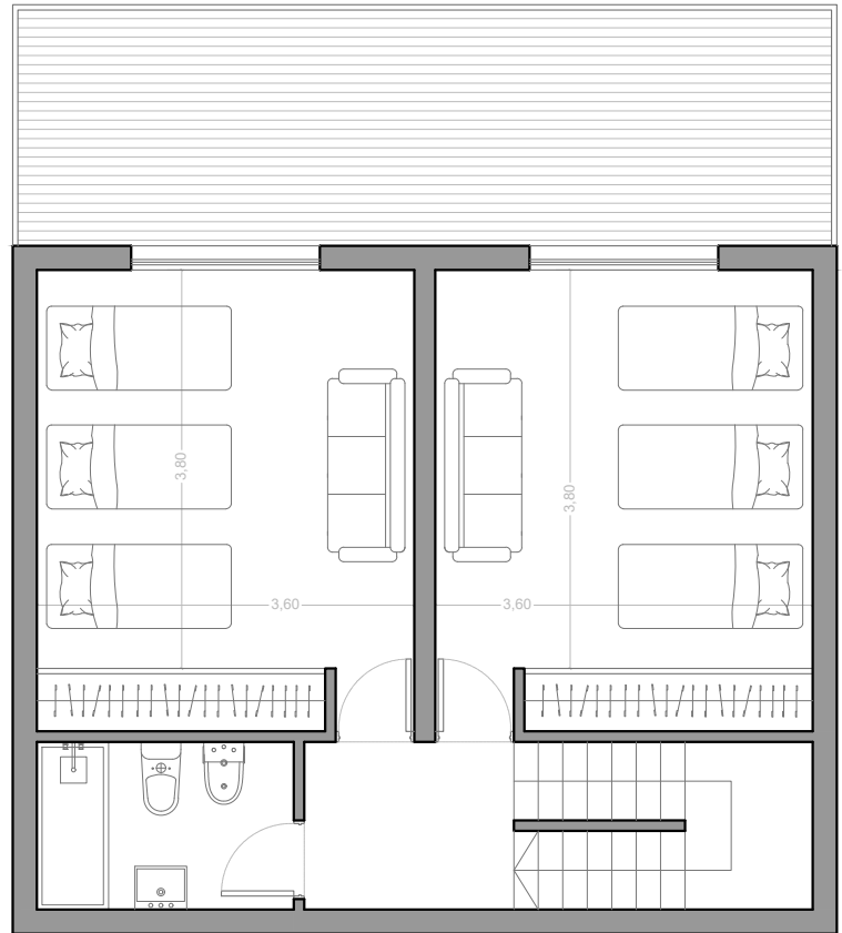
Planta Alta
